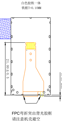
FPC弯折示意图 FPC展开出货
