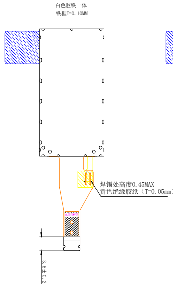
FPC弯折示意图 FPC展开出货
